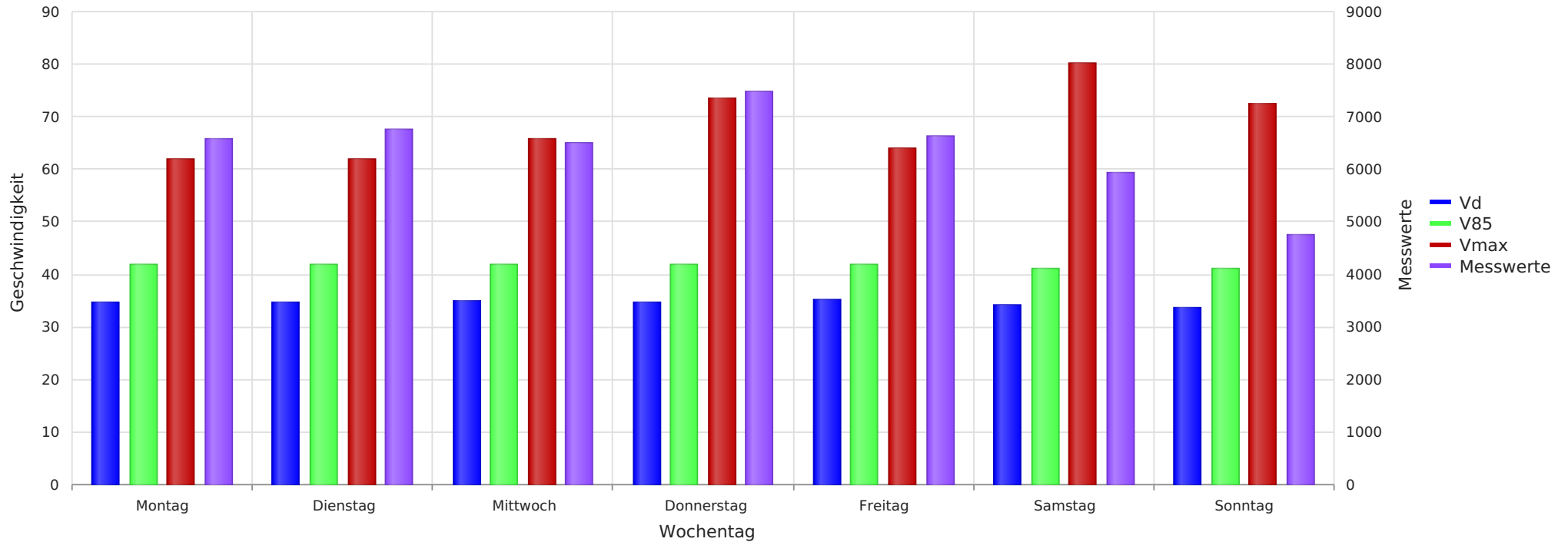
2023_06_12-07_03 Westerholzstraße 15 Richtung Ortskern Vd, V85, Vmax, Anzahl der Messwerte vs. Wochentag
