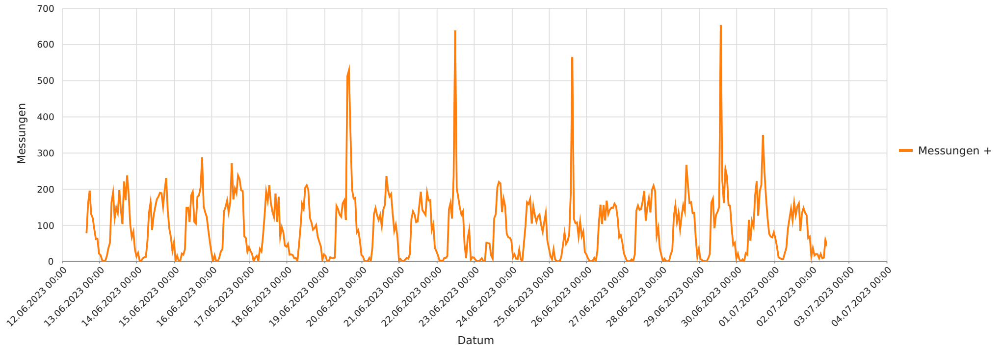
2023_06_12-07_03 Westerholzstraße 15 Richtung Ortskern Anzahl der Messwerte vs. Messzeitraum
