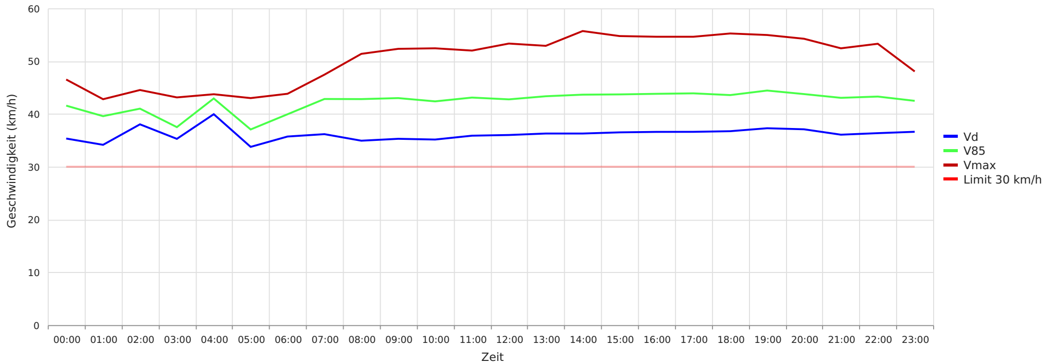
2023_06_12-07_03 Westerholzstraße 15 Richtung Ortskern Vd, V85, Vmax vs. Uhrzeit
