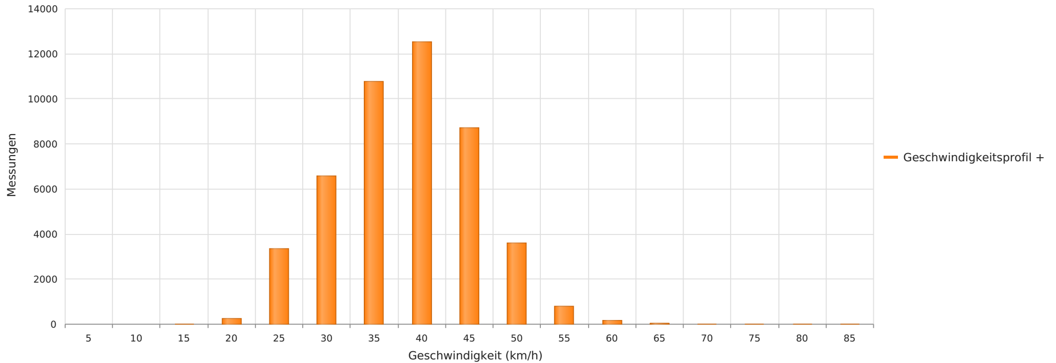
2023_06_12-07_03 Westerholzstraße 15 Richtung Ortskern Anzahl der Messwerte vs. Geschwindigkeit
