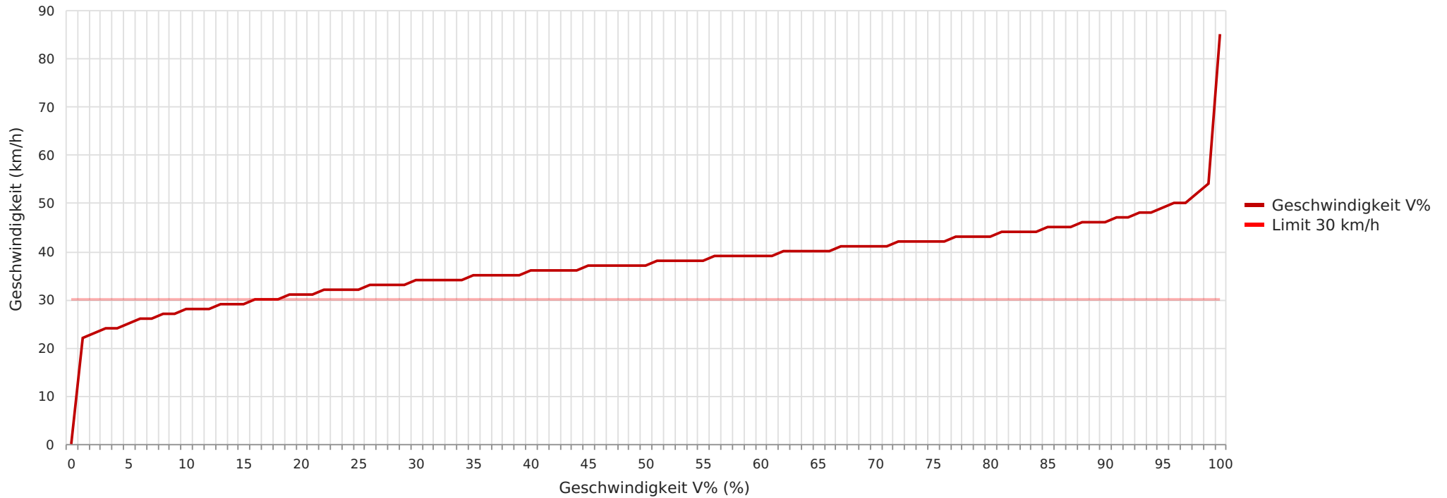
2023_06_12-07_03 Westerholzstraße 15 Richtung Ortskern Geschwindigkeit vs. prozentueller Anteil an Messwerten
