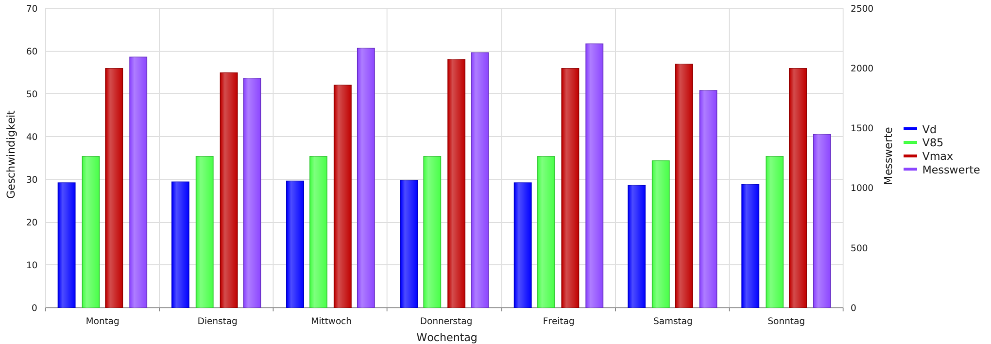
2023_05_09-16 Sprockhofer Str. 12 Richtung Ortskern Vd, V85, Vmax, Anzahl der Messwerte vs. Wochentag
