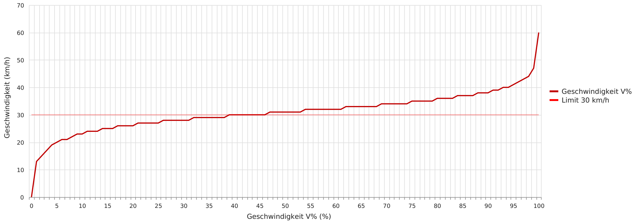
2023_05_09-16 Sprockhofer Str. 12 Richtung Ortskern Geschwindigkeit vs. prozentueller Anteil an Messwerten
