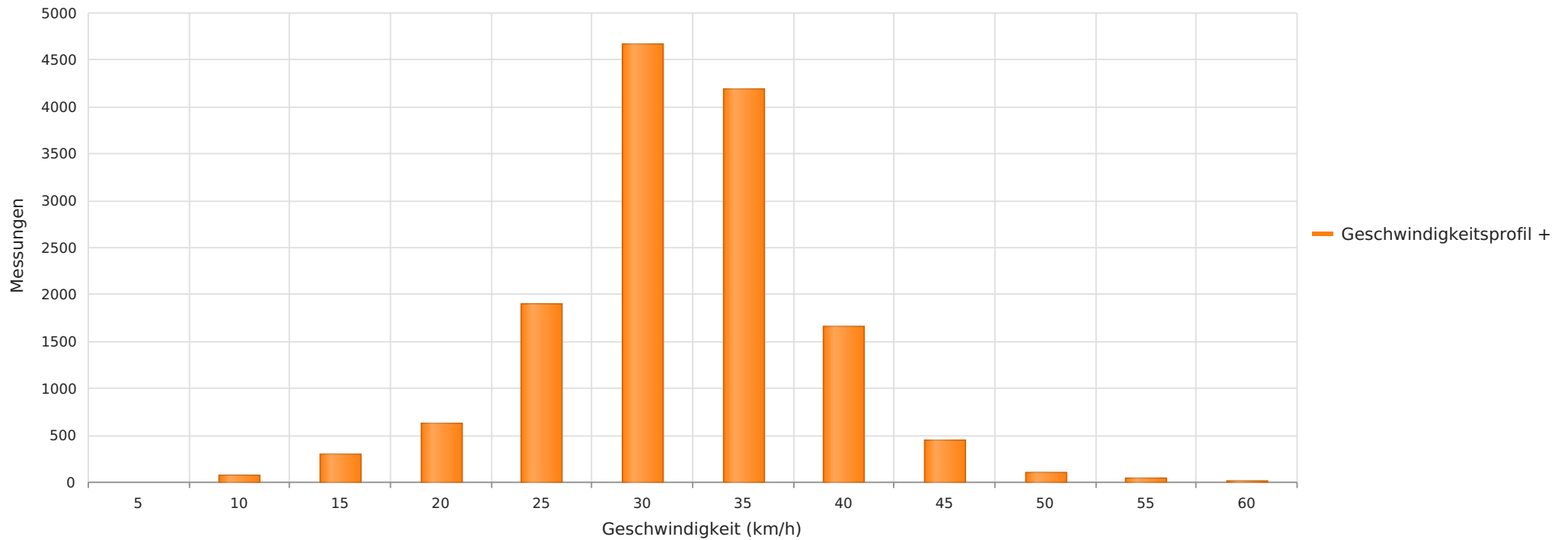
2023_05_09-16 Sprockhofer Str. 12 Richtung Ortskern Anzahl der Messwerte vs. Geschwindigkeit
