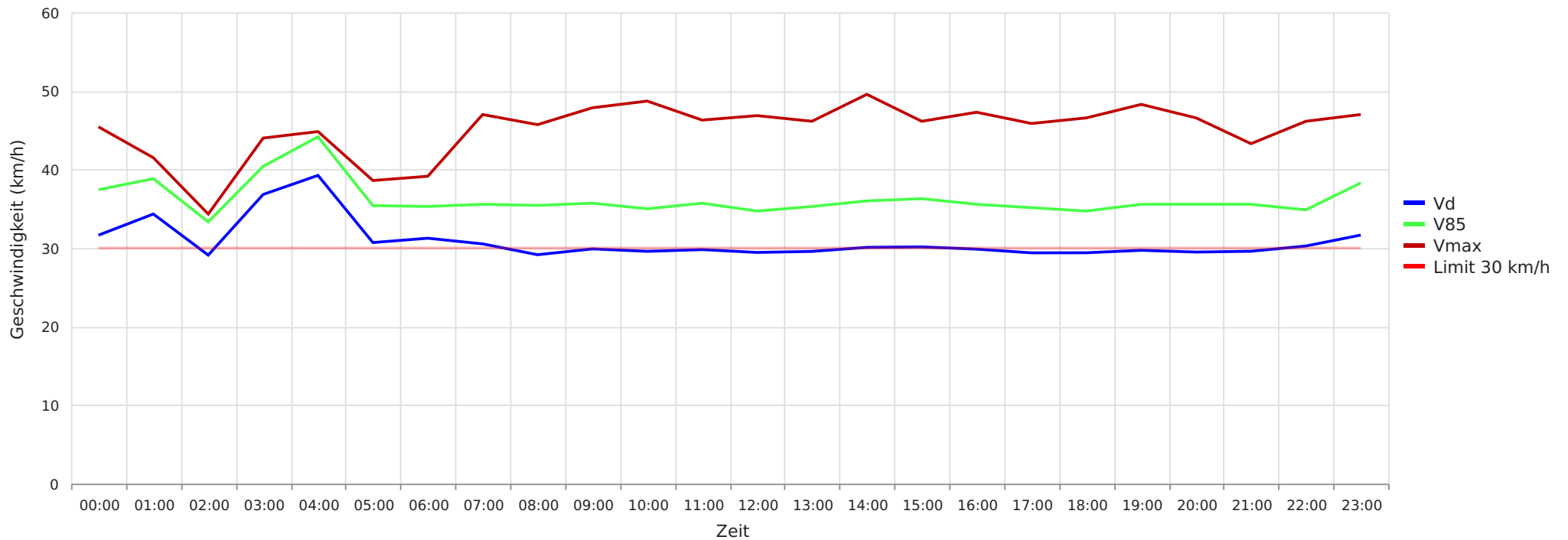
2023_05_09-16 Sprockhofer Str. 12 Richtung Ortskern Vd, V85, Vmax vs. Uhrzeit
